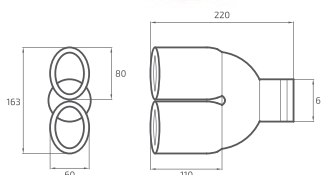
PONTEIRA DUPLA REF. 658.1-57D / 658.1-57E
