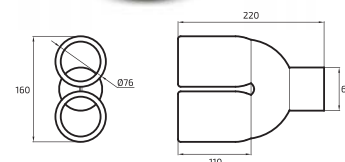
PONTEIRA DUPLA REF. 687.B1-60E
