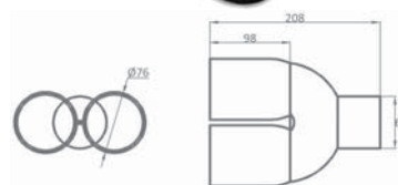
PONTEIRA DUPLA REF. 502B1-50
