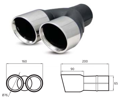
PONTEIRA DUPLA REF. 563.1-60
