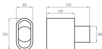
PONTEIRA DUPLA REF. 598.1-60
