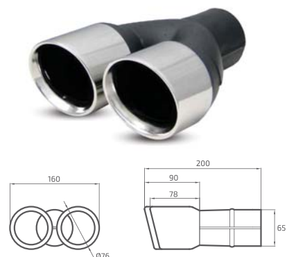
PONTEIRA DUPLA REF. 587.1-60ESQ
